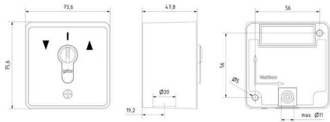
Aufbau-Schlüsselschalter Mit PHZ Art.: 110.13E2.10
