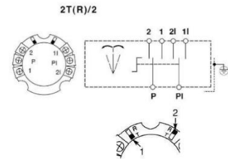
Aufbau-Schlüsselschalter Mit PHZ Art.: 110.13E2.10
